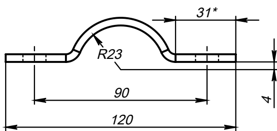
Поз.5 (Полухомут)
