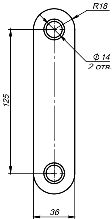
Поз.4 (Серьга)
