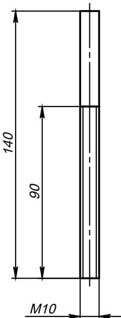
Поз.1 (Шпилька)
