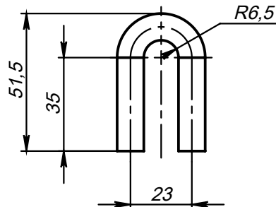
Поз.2 (Ушко)
